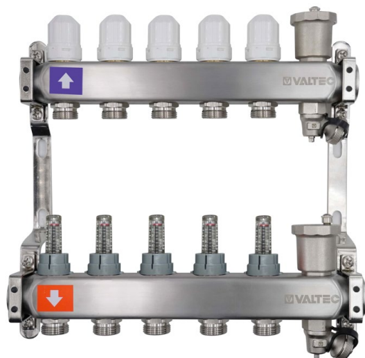
КОЛЛЕКТОРНЫЙ БЛОК ИЗ НЕРЖАВЕЮЩЕЙ СТАЛИ С РЕГУЛИРУЮЩИМИ КЛАПАНАМИ И РАСХОДОМЕРАМИ
