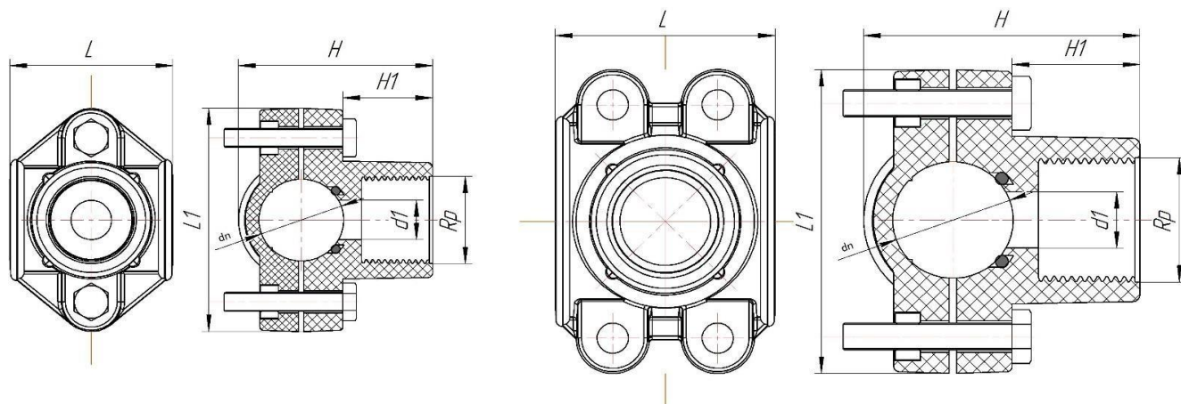
Рисунок 2. Седелка отводная. Габаритные и присоединительные размеры
