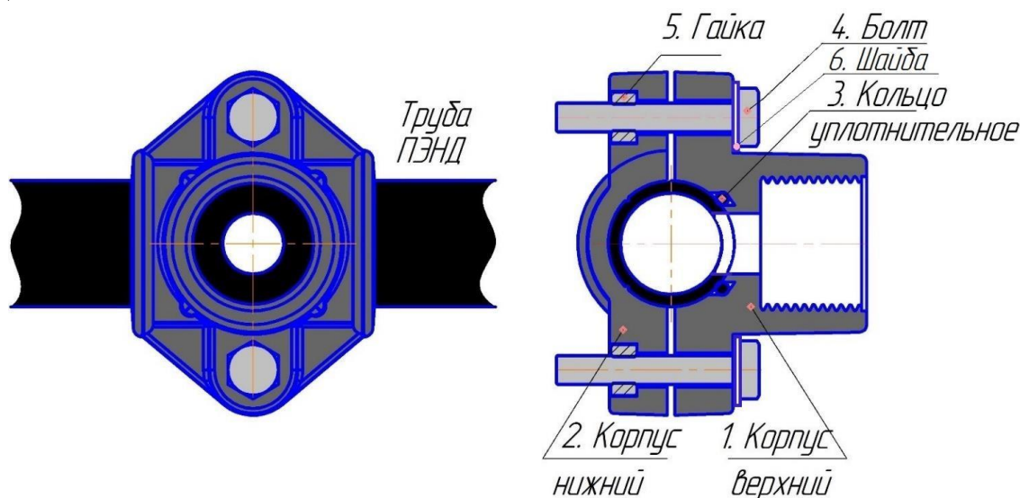
Рисунок 1. Конструкция седелки
